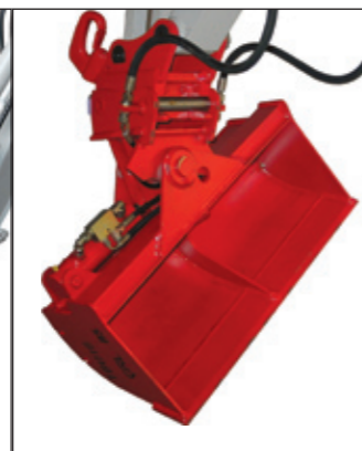
Hydraulisch schwenkbarer Grabenräumlöffel
